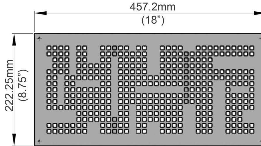
TOP scale 1:4
